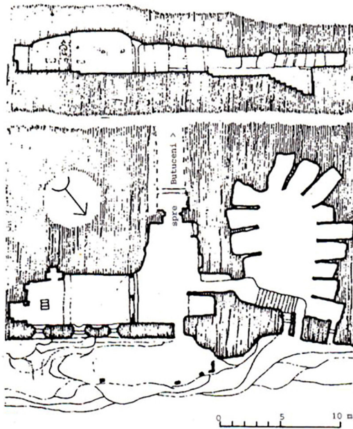
Fig. nr. 9. Plan și secțiune longitudinală a complexului monahal de la Butuceni.
