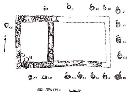
Fig. nr. 1. Planul arheologic cu urme de zid și baze de coloane al edificiului de piatră de la Sobari (Soroca), după Niculiță, Popa.
